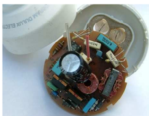
Fot. 3 Elektroniczny układ zapłonowy świetlówki komp.
