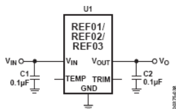
Rys. 4 Schemat podłączenia układu REF01C jako źródła napięcia referencyjnego 10.00V
