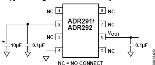
Rys. 3 Schemat podłączenia układu ADR292 jako źródła napięcia referencyjnego 4.096V
